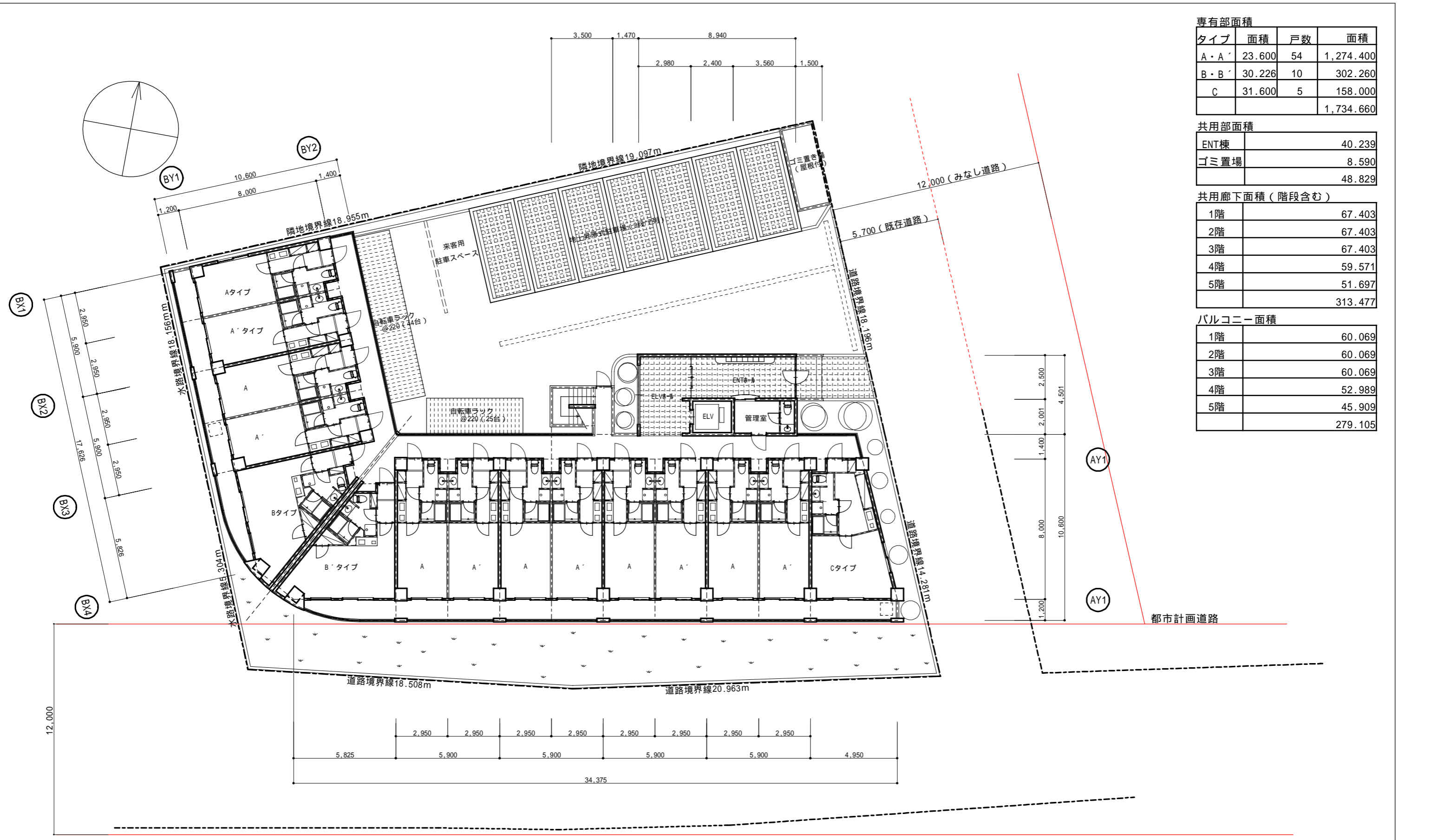
1階平面図、及び配置図 (S=1/200)
